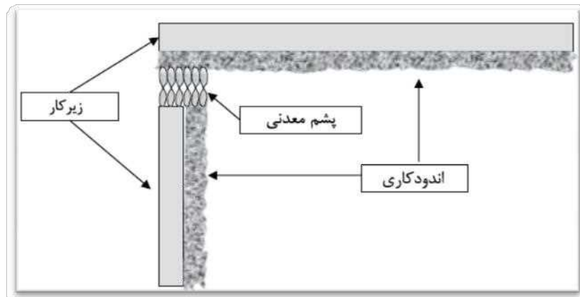
شکل الف-۱: الگوی درز قائم برای آزمون یک سیستم اندودکاری
