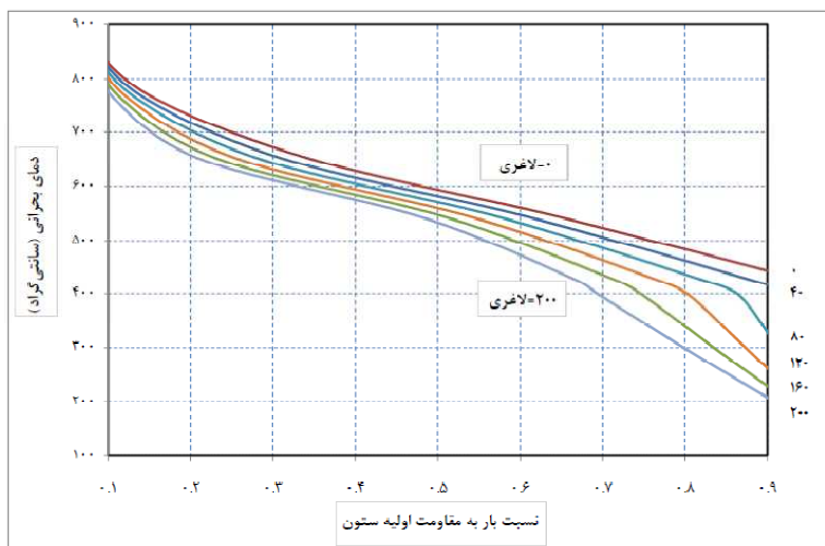
شکل ۱-۱۵: دمای بحرانی ستون با فولاد ST37 برای لاغری‌ها و نسبت‌های مختلف بار فشاری وارده به
