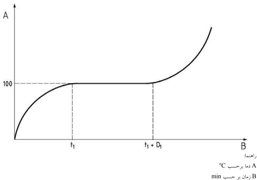
شکل ۴-ث-۴ معرفی رطوبت پایدار
