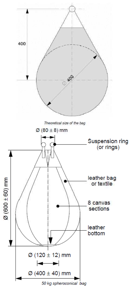
شکل ۳-۱: ضربه زننده جسم نرم
