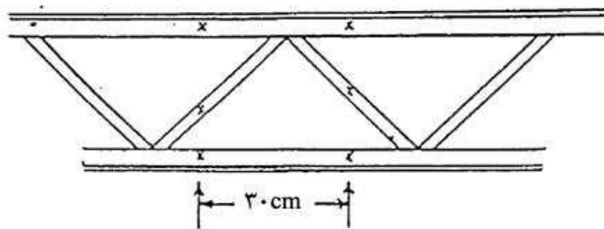
شکل ۴-ب-۴ مکان‌های اندازه‌گیری ضخامت مواد محافظ در برابر حریق بر روی تیرچه‌ها (خرپاها)
