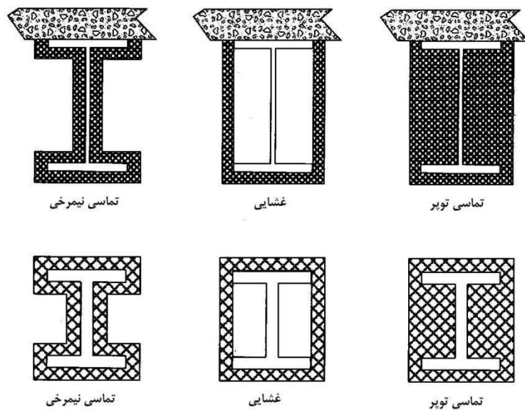
شکل ۱-۳: انواع محافظت تماسی و غشایی
