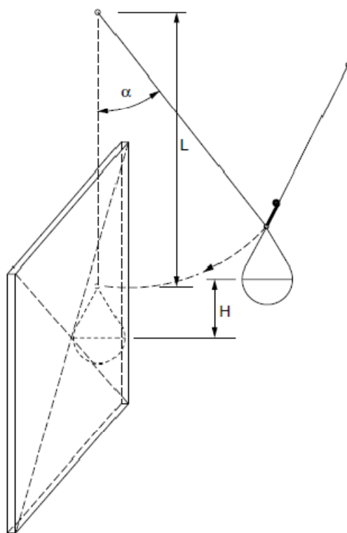
شکل ۳-ث ۲-ضربه بر روی مجموعه قائم
