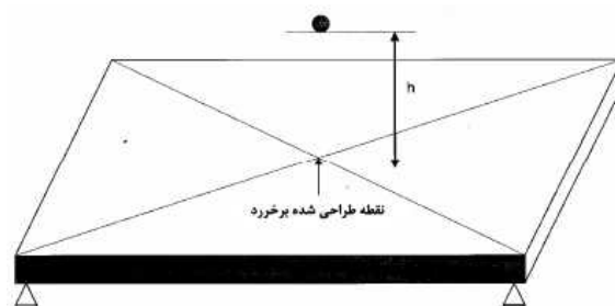
شکل ۳-۴ مجموعه آزمایشگاهی برای آزمون ضربه جسم سخت
