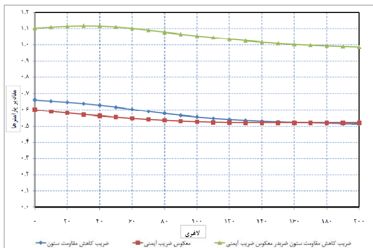
شکل ۱۰-۱: کنترل گسیختگی ستون با فولاد ST37 مطابق آئین نامه EN 1993-1-2 در دمای ۵۳۸°C
