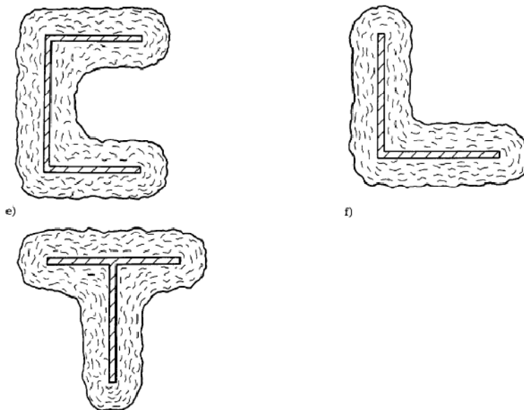
شکل ۵-۲- محصور کردن و پروفیل‌ها با شکل داخل‌شونده
